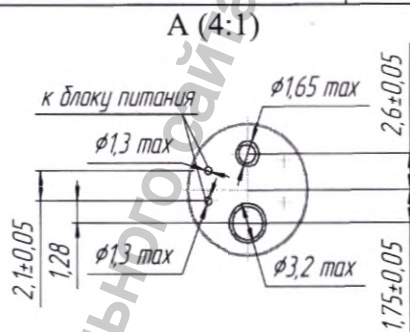
Рисунок 2 – Наконечник стоматологический турбинный с подсветкой НСТкc-300-«TM»-M4
