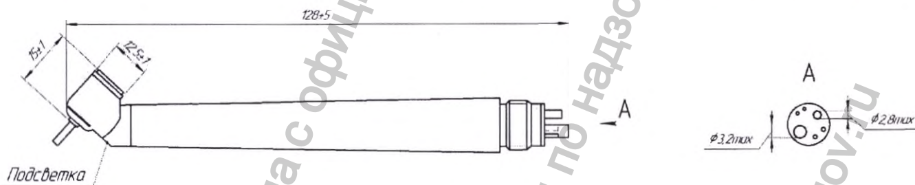
Рисунок 2 – Наконечник стоматологический турбинный с подсветкой НСТкc-300-«TM»-M4
